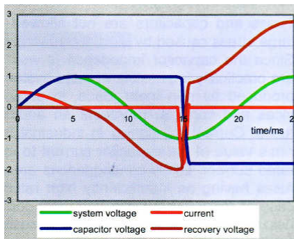
شکل ۱۰،۱۸- دیگرام قطع خازنی
