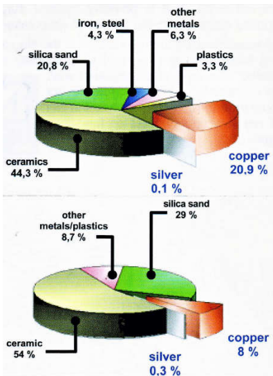
شکل ۲۳،۱ – مواد تشکیل دهنده المان فیوز
