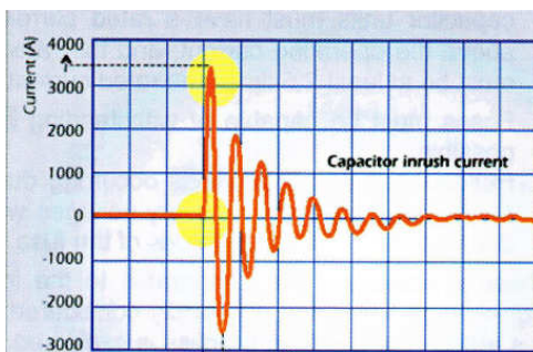
شکل ۱۰،۱۶ - جریان هجومی خازنی
